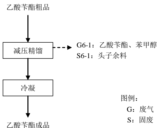
图4.1-8 乙酸苄酯生产工艺流程图
