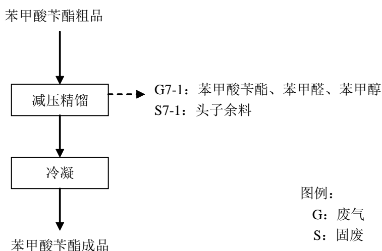
图4.1-9 苯甲酸苄酯生产工艺流程图
