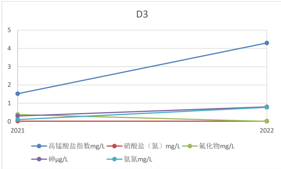
图8-3 D3点位污染物浓度变化趋势
