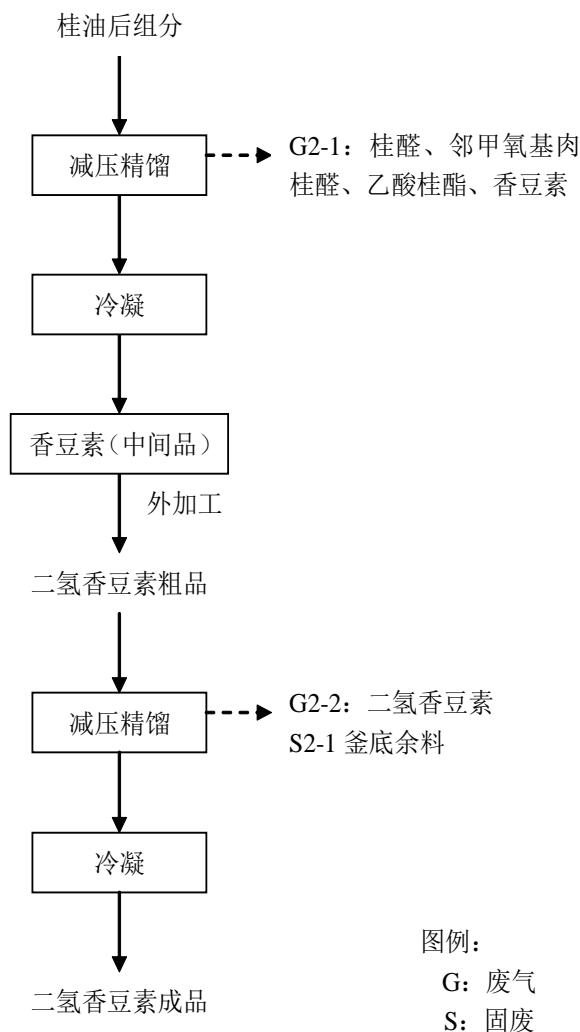
图4.1-4 二氢香豆素生产工艺流程图
