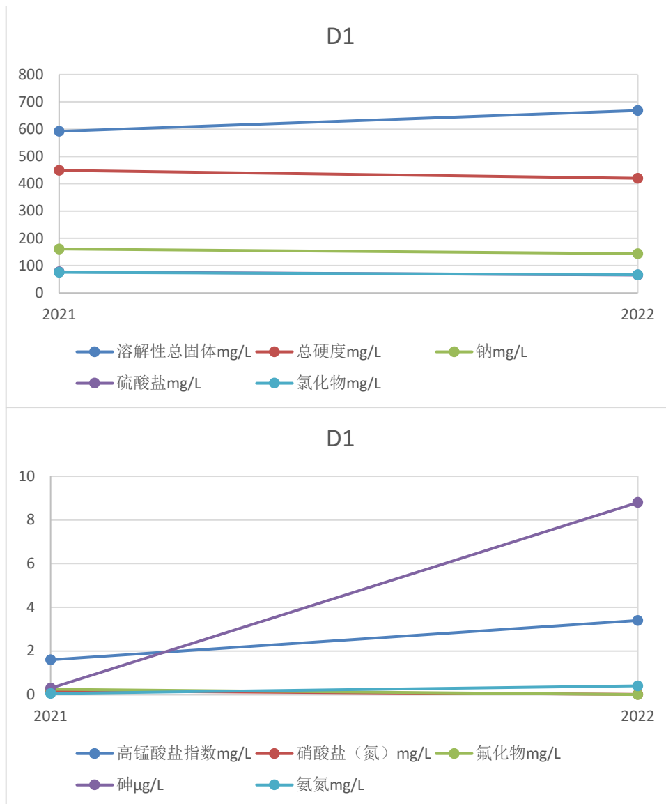
图8-1 D1点位污染物浓度变化趋势
